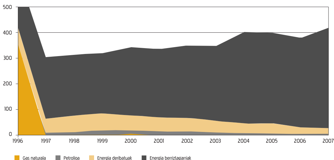
1.4.5. Grafikoa. Oinarritzko energiaren produkzioa (Ktep)
